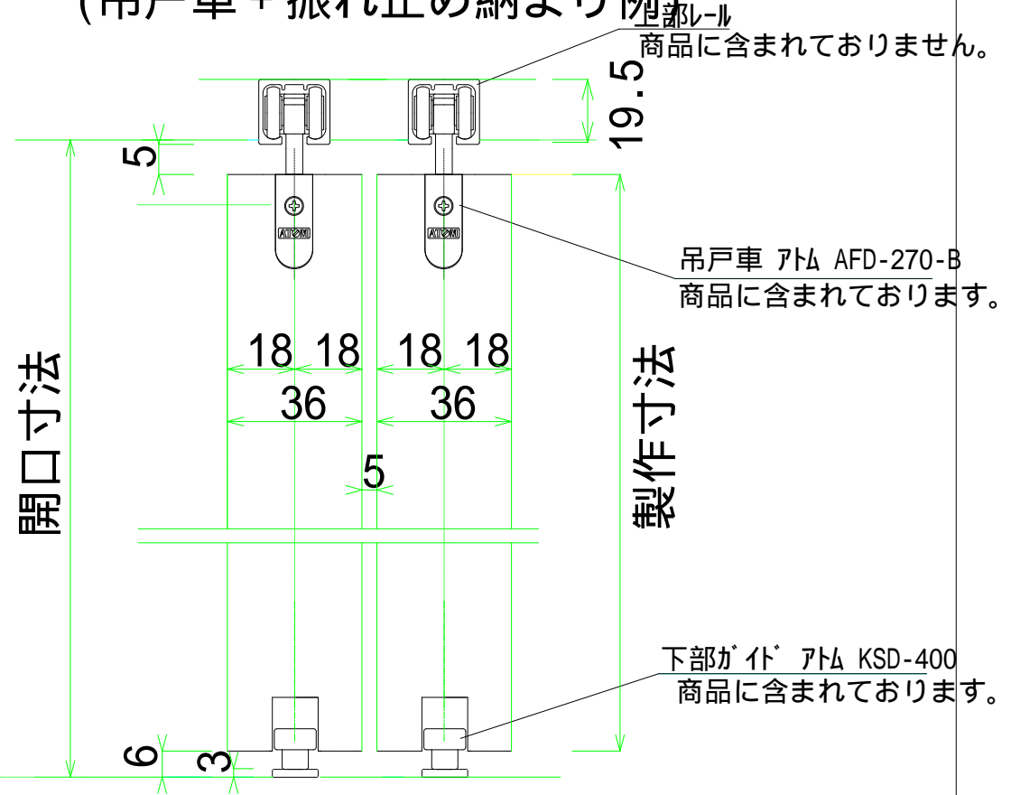
(吊戸車 + 振れ止め納まり例)
