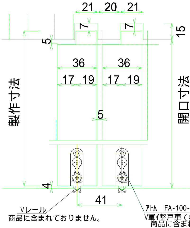
(戸首 + レール納まり例)
